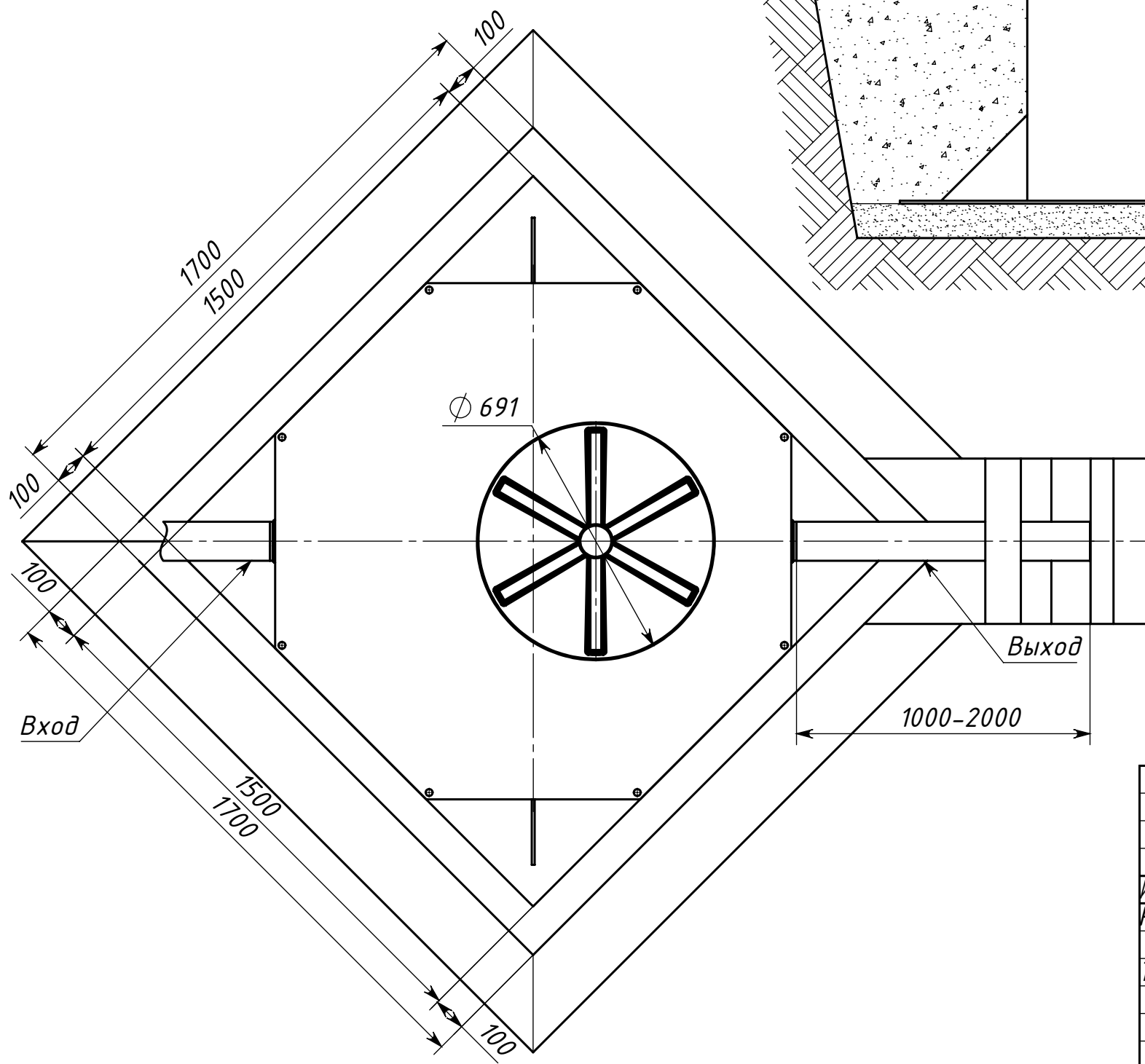
Вид сверху
